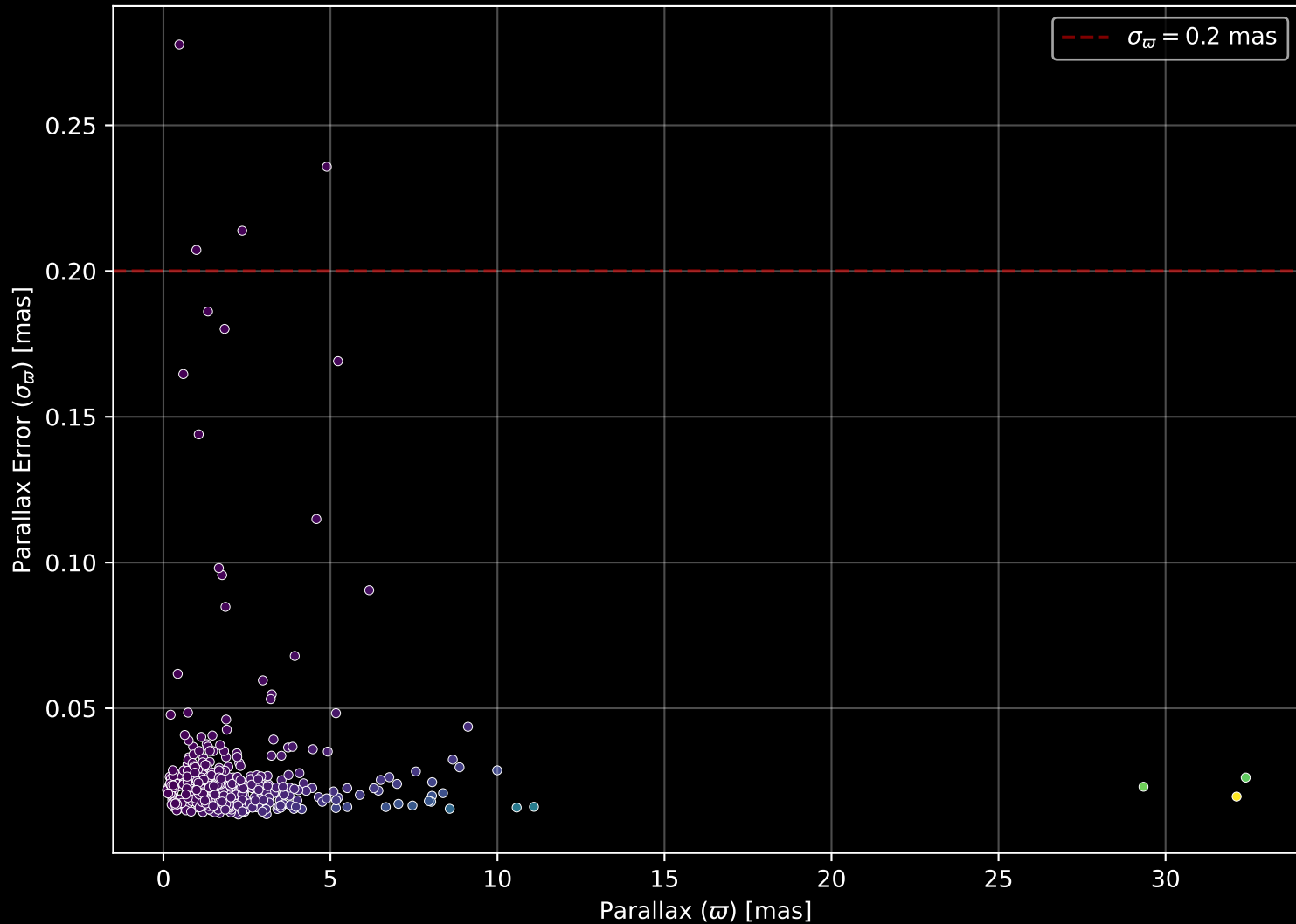
GALAH DR4 Field: [6590] Parallax Quality (n= 452)
