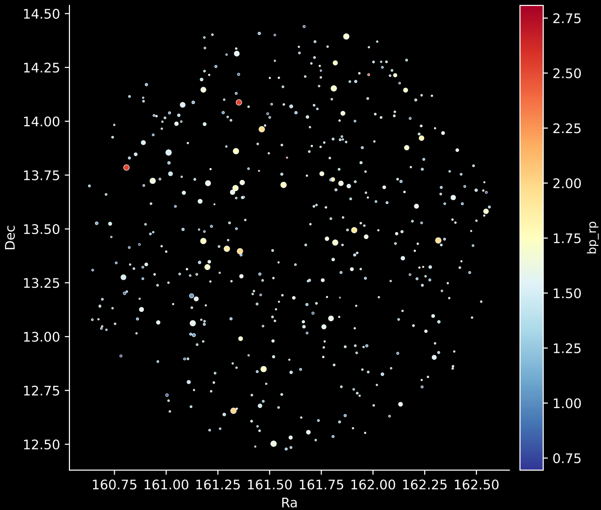
GALAH DR4 Field: [6590] Stars: 452
