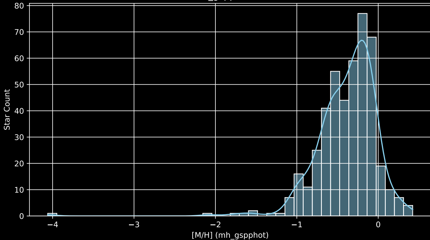
GALAH DR4 Field: [6590] [M/H] (mh_gspphot) (n= 451)
