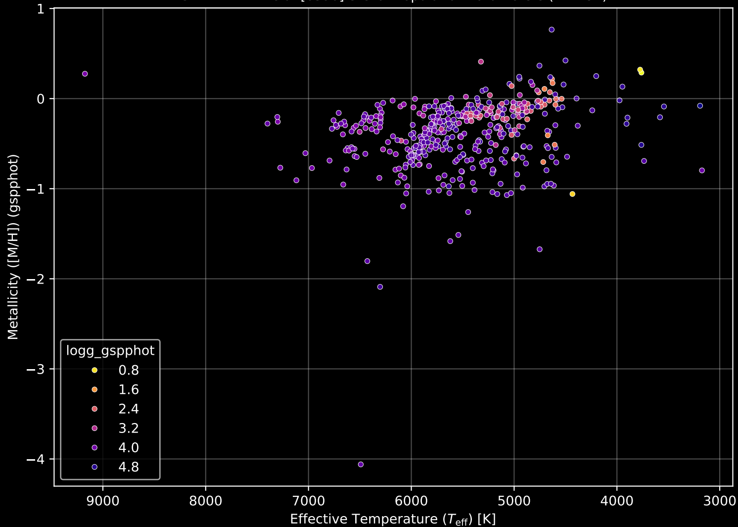
GALAH DR4 Field: [6590] Stellar Population Parameters (n= 452)
