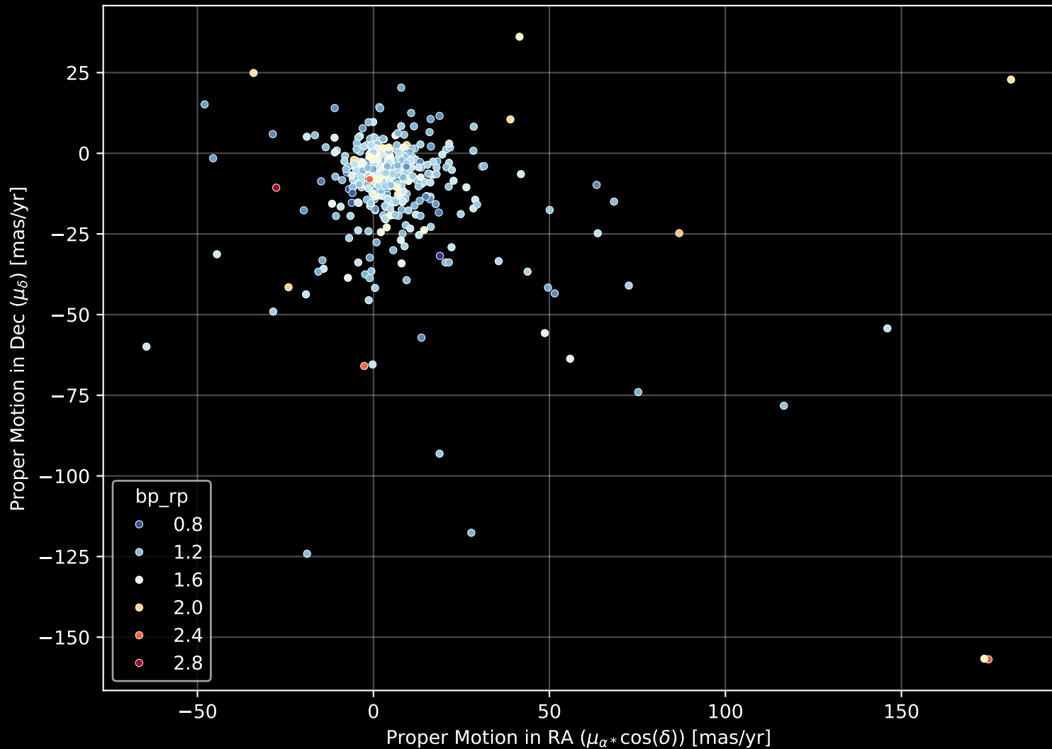
GALAH DR4 Field: [6590] Proper Motion Diagram (n= 452)
